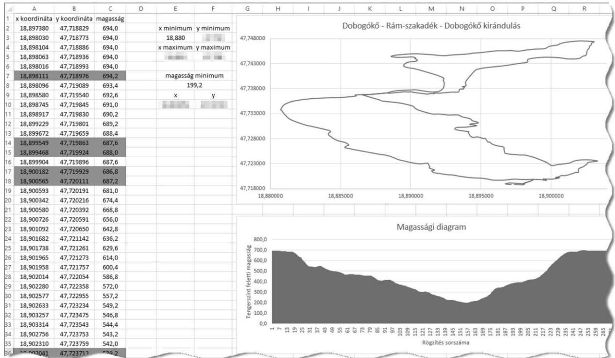
nyomvonal munkalap
